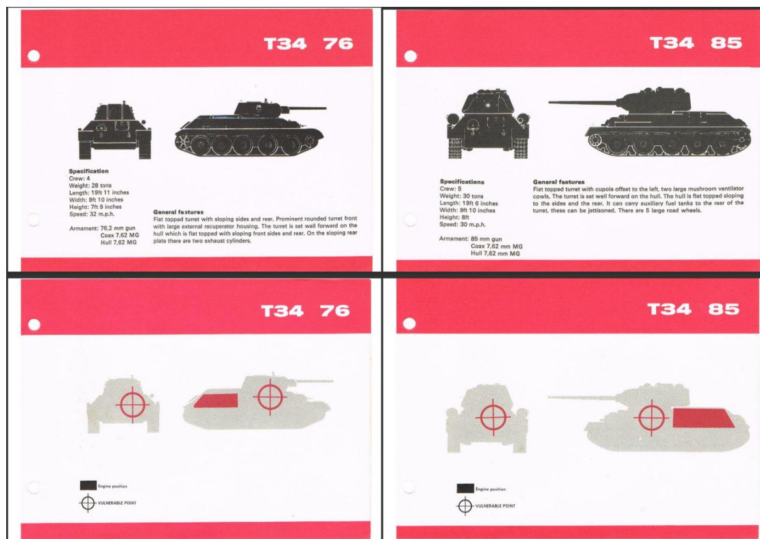
Рис. 5. Советские танки Т-34-76 и Т-34-85
