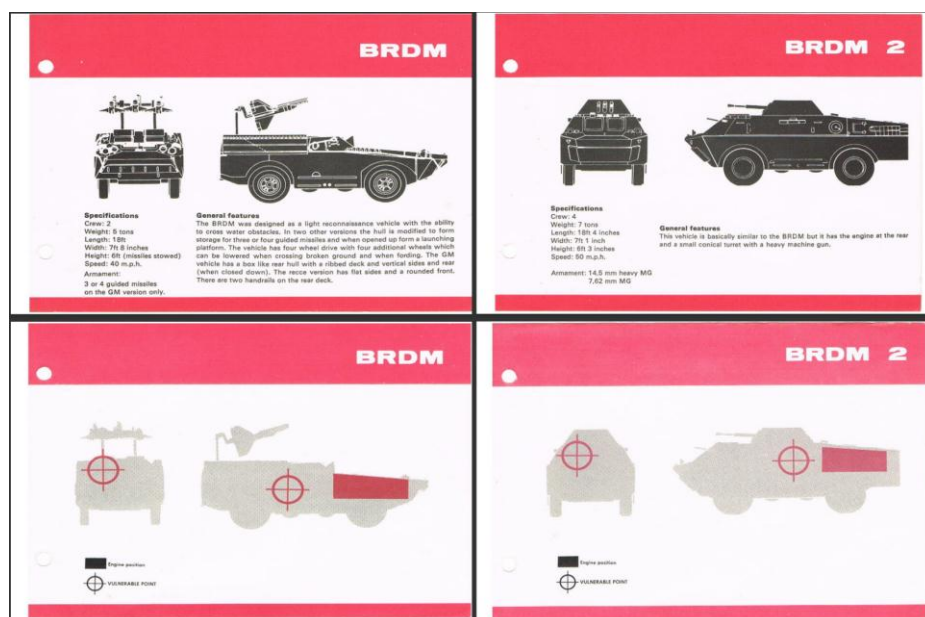
Рис. 4. Советские БРДМ и БРДМ-2
